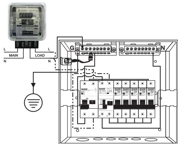
การต่อสายโดยการใช้ MCB เป็นเมนร่วมกับ RCDs
