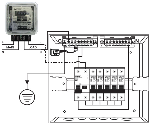
การต่อสายโดยการใช้ MCB 2P เป็นเมน
